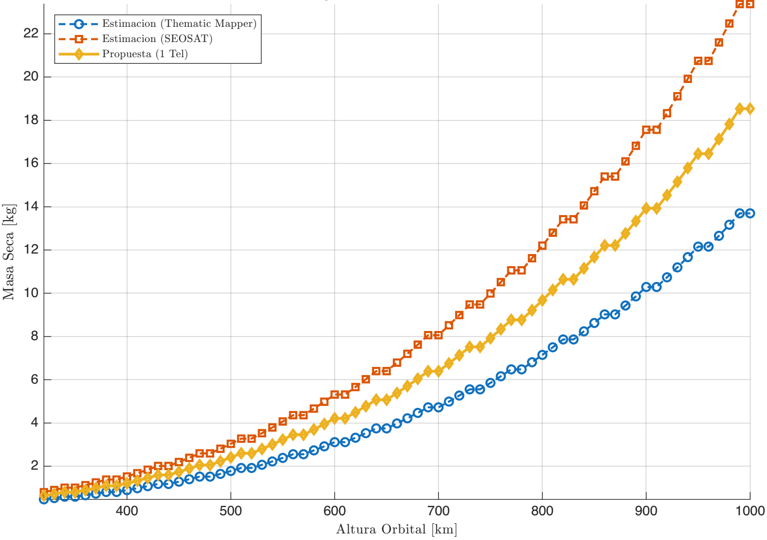
Comparativa de Masa Seca vs. Altura Config: 3 Sat, 1 Tel, Det 2, Korsch
